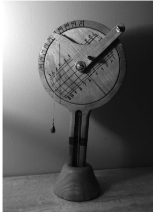
Cadran de hauteur réalisé par Richard Frenette sur son tour à bois.
