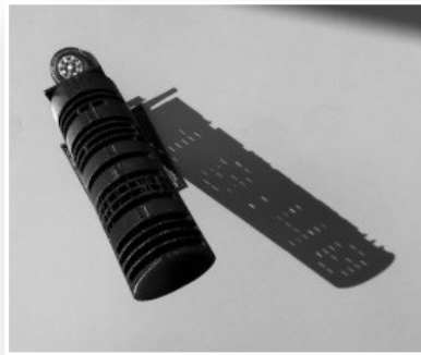
Cadran solaire utilisant les technologies actuelles : fabriqué avec une imprimante 3D. Il permet de projeter sur une surface plane l'indication de l'heure solaire sous forme numérique. (Photo Roger Torrenti)
