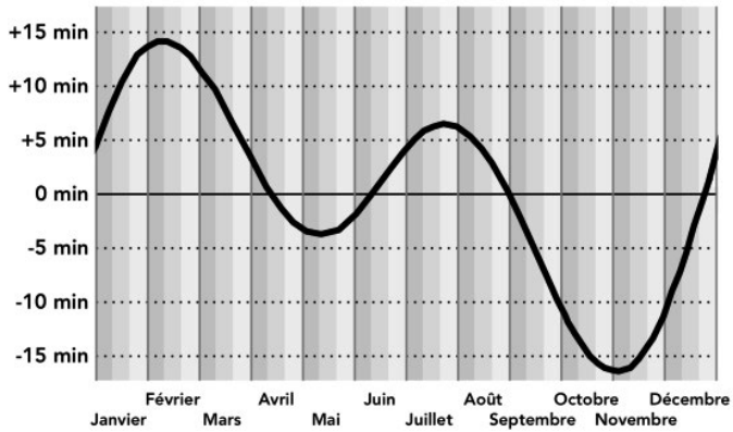
Courbe de l'équation du temps. (Illustration Roger Torrenti)
